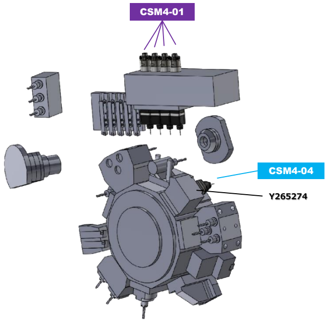
•Cincom L20Ⅷ·Ⅸ·Ⅹ·Ⅻ
