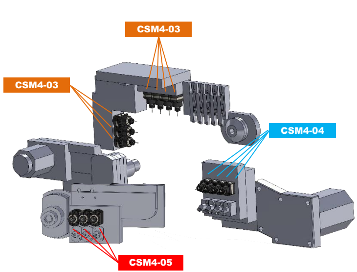
•Cincom L20Ⅷ·Ⅸ·Ⅹ·Ⅻ
